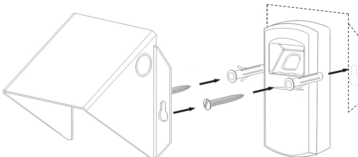
Рисунок 2 – Монтаж козырька
