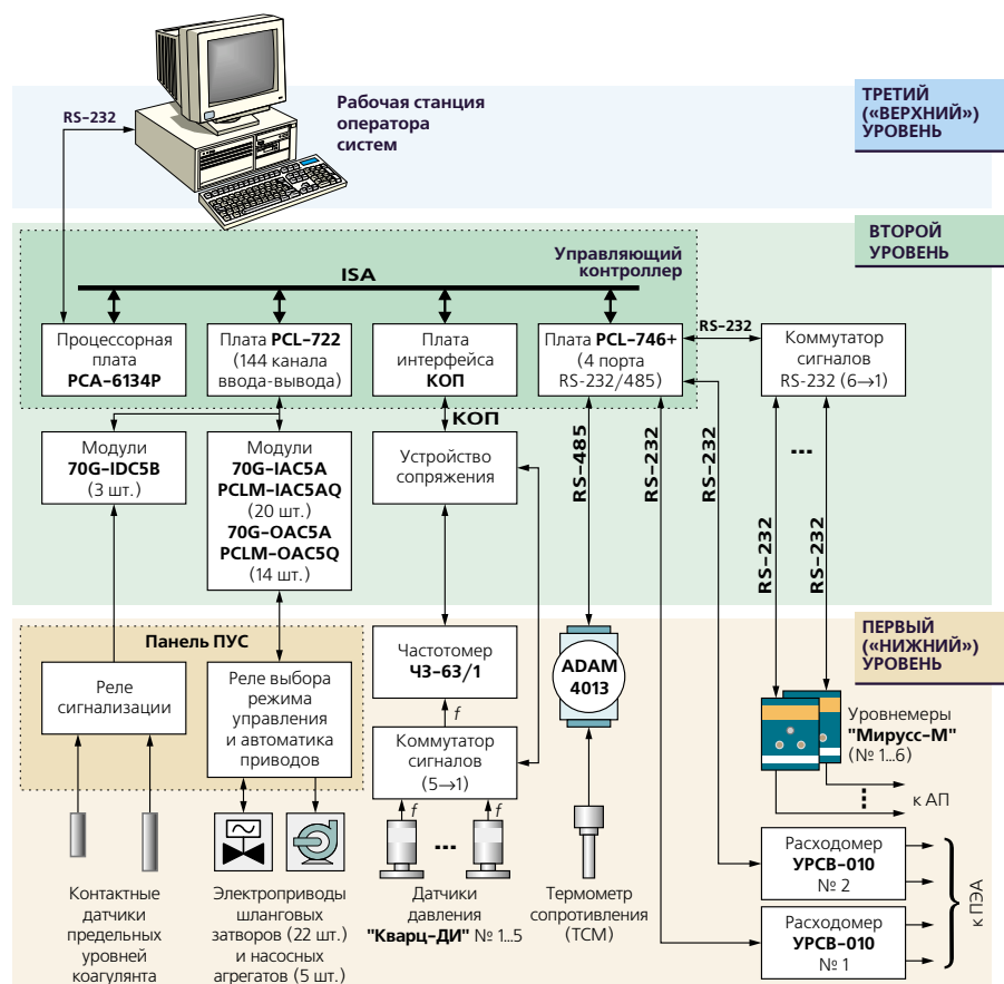
Рис. 2. Структурная схема СИПК и СПДК
