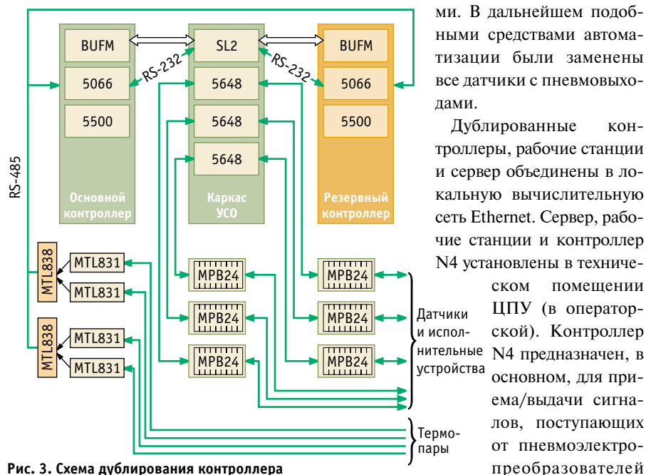
Рис. 3. Схема дублирования контроллера
