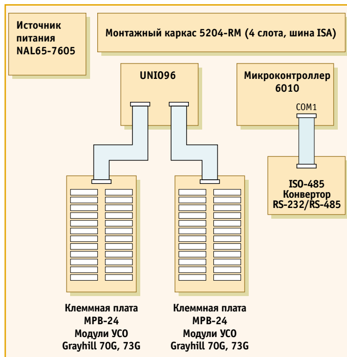
Рис. 3. Структура контроллера ГУВ
