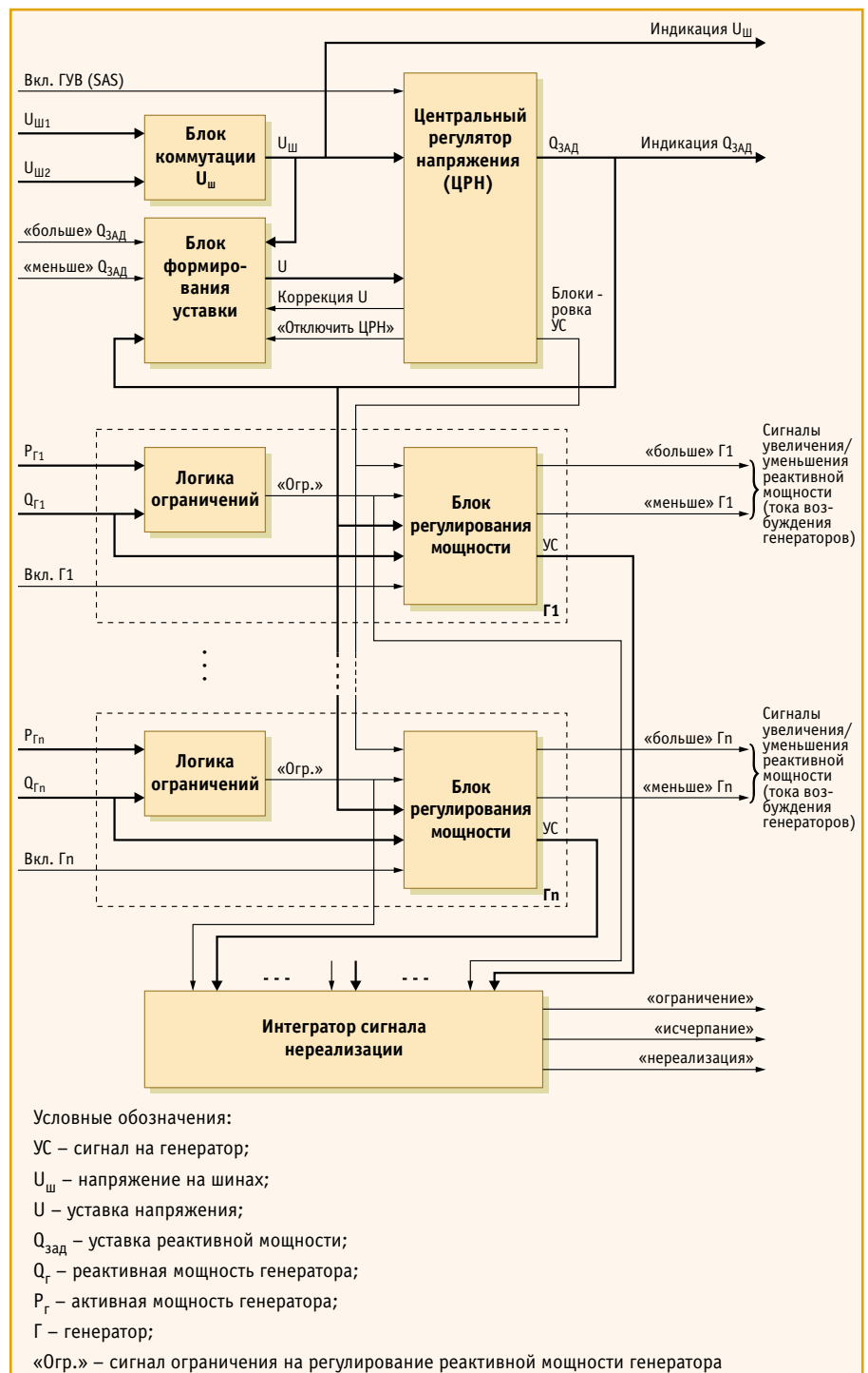
Рис. 2. Упрощенная структурная схема одного контура регулирования
