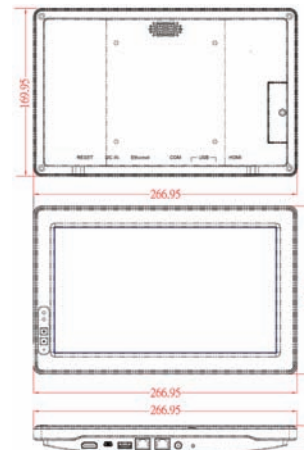
IPPC10A5-RE Dimensions
