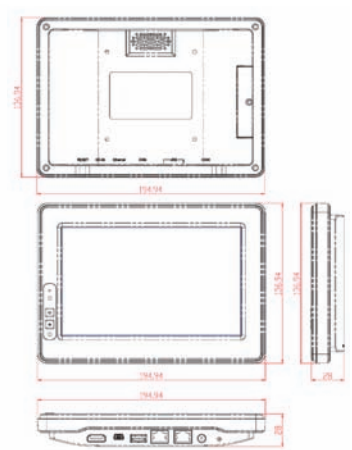
IPPC07A5-RE Dimensions
