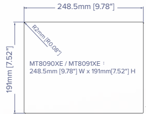
Cutout Dimensions
