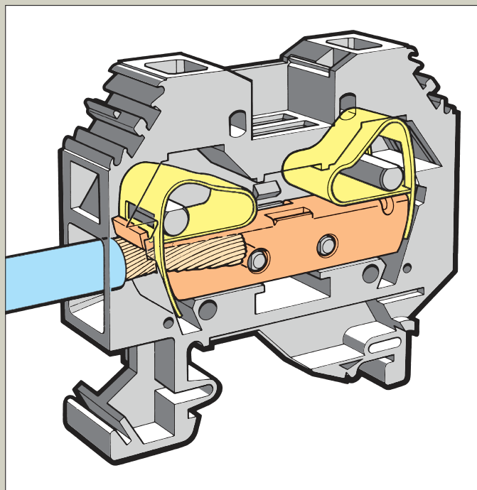
Подключение проводников
