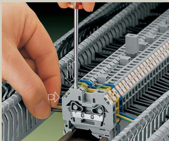
Подключение проводников
