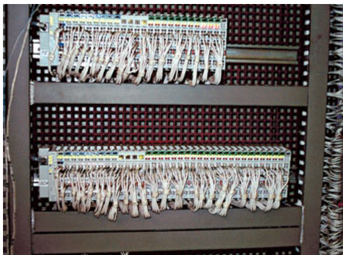
Рис. 2. Контроллеры (основной и резервирующий) WAGO I/O-System серии 750
