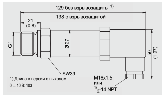
Измерительный преобразователь 7MF1564-... с подключением к процессу G1" (внешняя), монтаж заподлицо, размеры в мм
