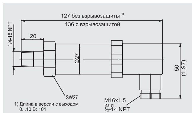
Измерительный преобразователь 7MF1564-... с подключением к процессу 1/4"-18 NPT (внешняя), размеры в мм
