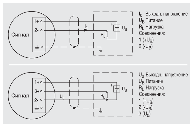
Преобразователь давления SITRANS P, серия Z (7MF1564-...), схема подключения, с токовым выходом (вверху) и выходом напряжения (внизу)
