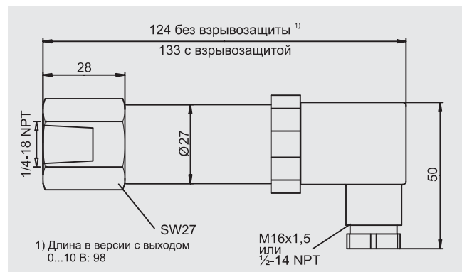
Измерительный преобразователь 7MF1564-... с подключением к процессу 1/4"-18 NPT (внутренняя), размеры в мм
