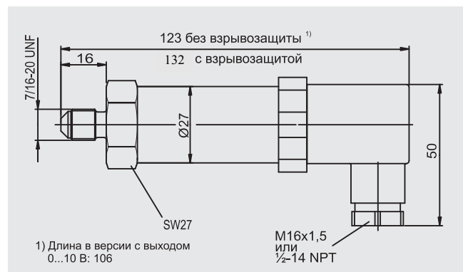
Измерительный преобразователь 7MF1564-... с подключением к процессу 7/16-20 UNF (внешняя), размеры в мм
