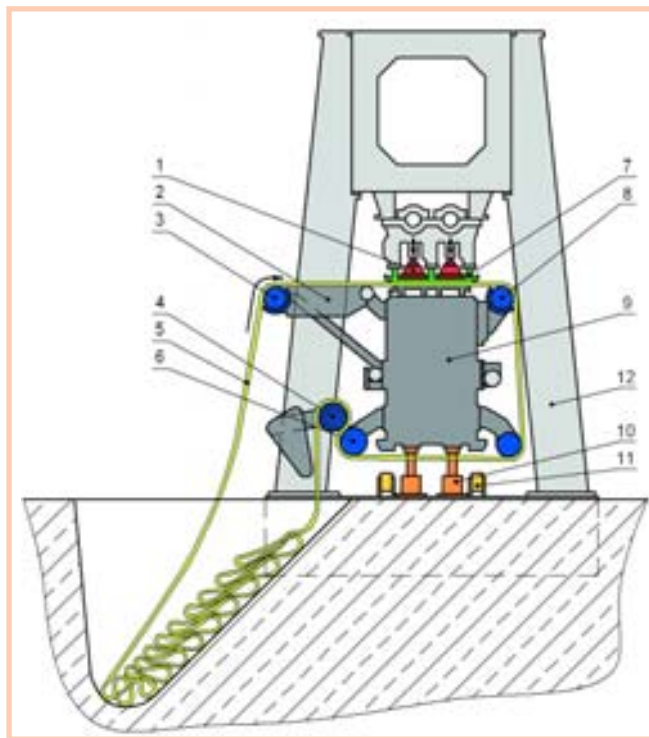
Условные обозначения: 1 — игельные брусья; 2 — стол подачи; 3 — тормозной вал; 4 — прижимной вал; 5 — полотно; 6 — тянущий вал; 7 — съёмник; 8 — выпускной вал; 9 — нижний брус; 10 — домкрат; 11 — ролик; 12 — станина.
