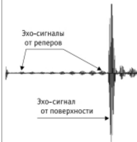
Рис. 2. Вид эхо-сигнала уровнемера
