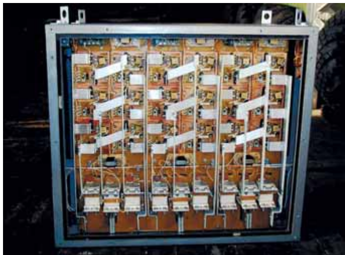
Рис. 3. Шестиканальный управляемый выпрямительный модуль (УВМ)
