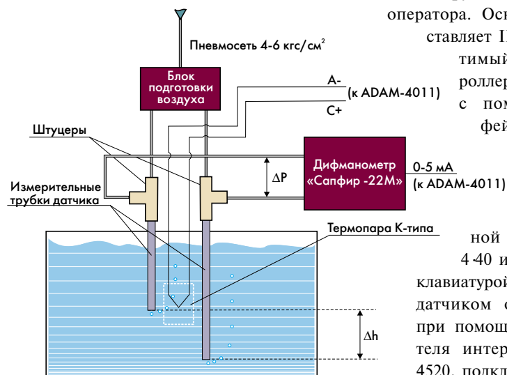
Рис. 2. Принцип работы датчика концентратомера
