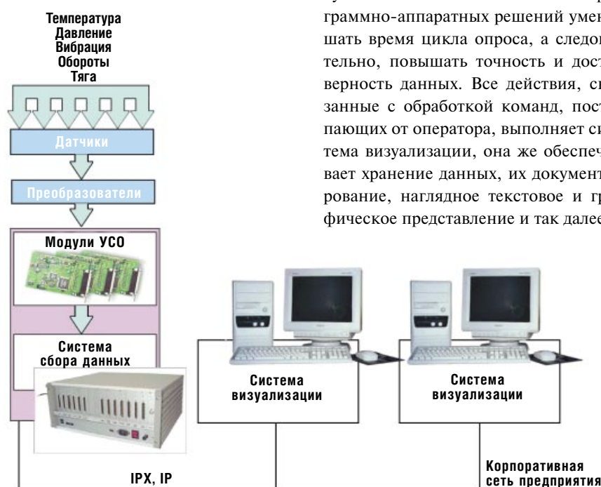
Рис. 1. Структурная схема АСКИ
