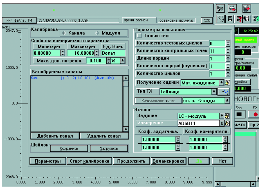
Рис. 6. Окно режима калибровки канала измерения термоздс
