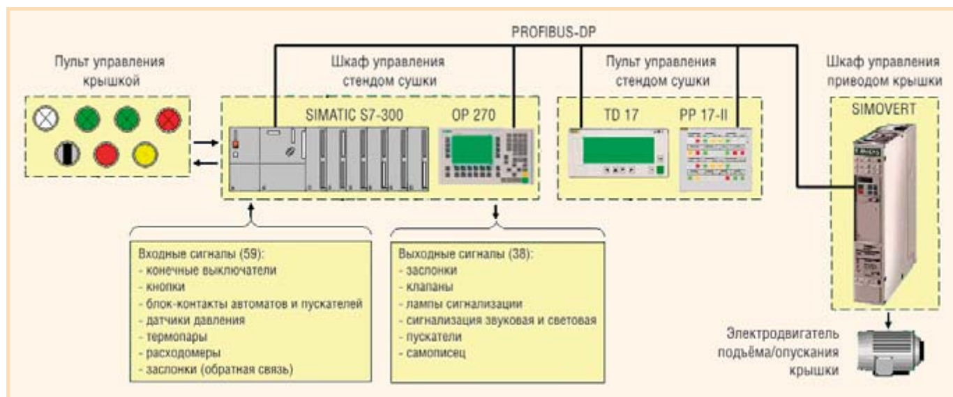
Рис. 3. Структурная схема системы управления станком сушки стальных ковшевых
