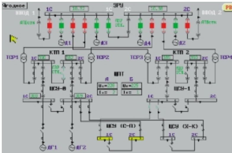
Рис. 14. Фрагмент схемы АСУ ТП электротехнического оборудования
