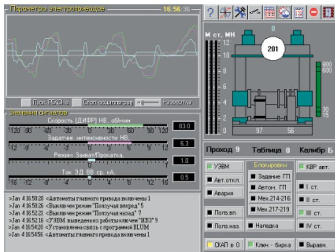
Рис. 10. Копия экрана программы визуализации параметров электроприводов
