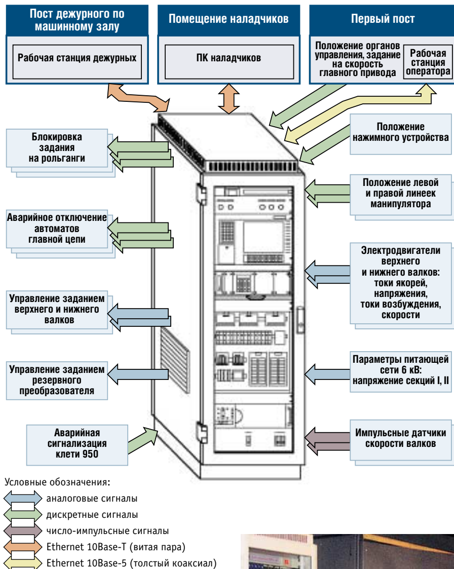
Рис. 4. Структурная схема системы управления клетью 950
