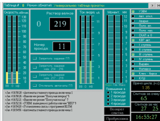
Рис. 11. Копия экрана программы оператора клетки 950
