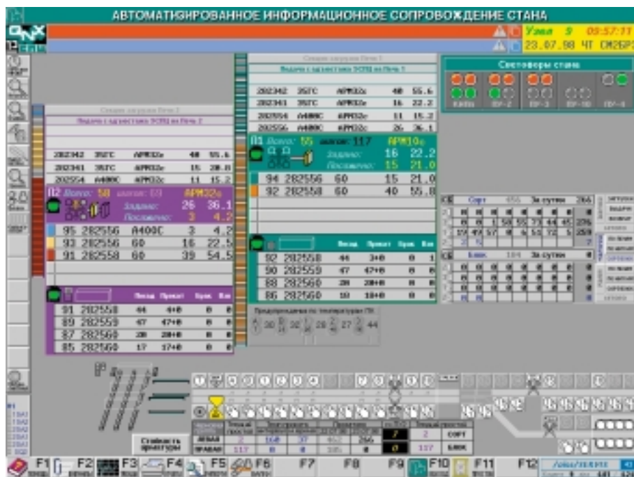
Рис. 6. Главная панель операторской станции поста станa, созданная в RTWin
