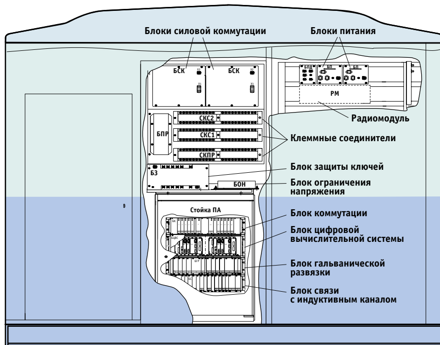
Рис. 3. Размещение полуконструкта ПА в головном вагоне
