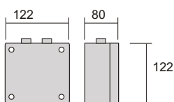
Exi data cable
