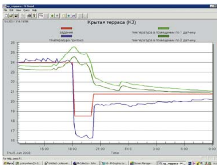
Рис. 4. Экранная форма отображения диаграммы комфортности из приложения M-Trend
