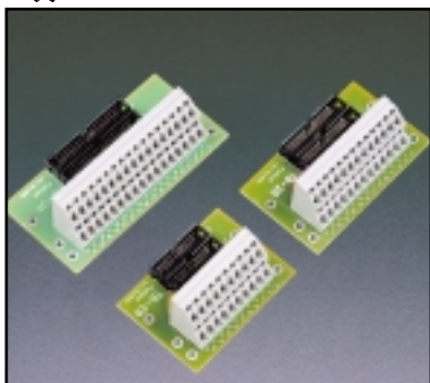
Клеммные платы ТВ-10/ТВ-20/ТВ-26/ТВ-34
