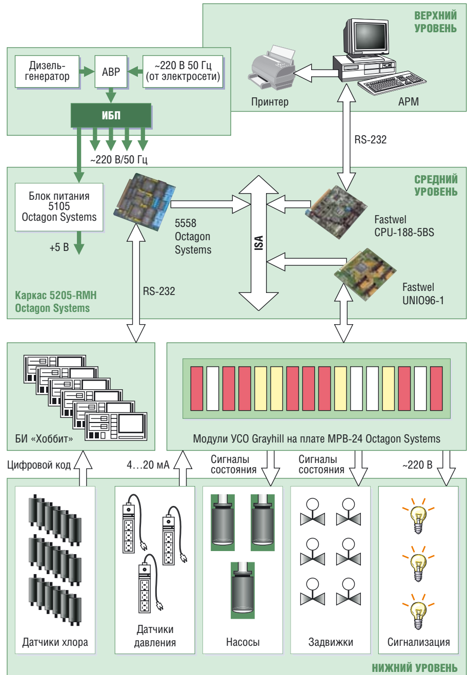
Рис. 3. Структурная схема АСУ ВЗ
