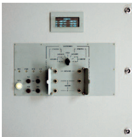
Рис. 9. Контроллер электрогидропривода
