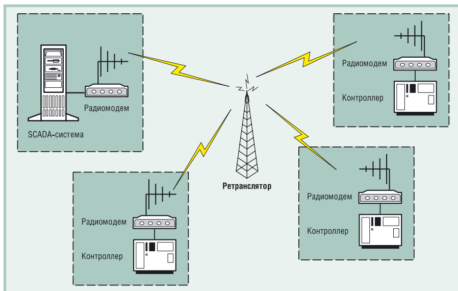
Рис. 3. Использование ретранслятора
