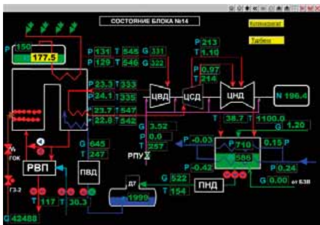
Рис. 4. Динамическая мнемосхема
