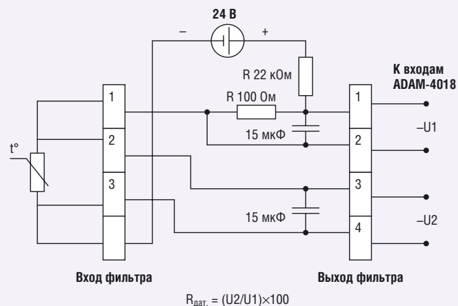
Рис. 8. Схема включения термометров сопротивления
