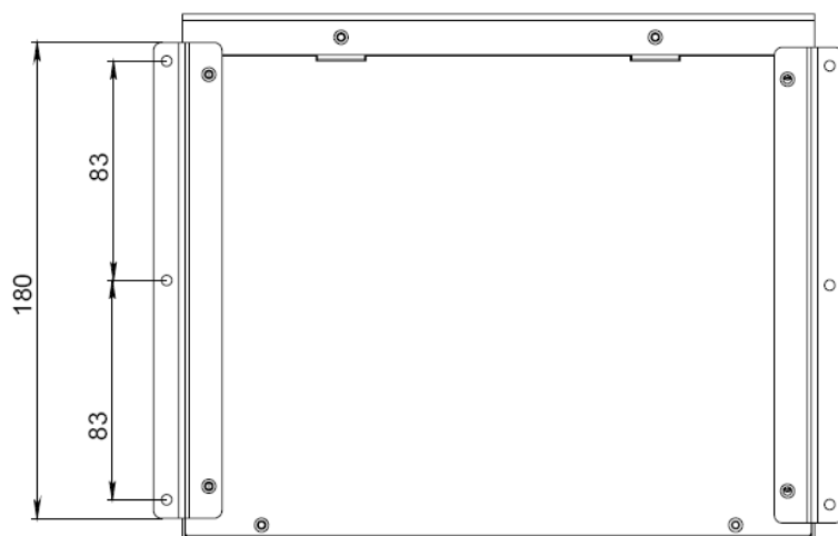
вид спереди: версия с 4 LAN
