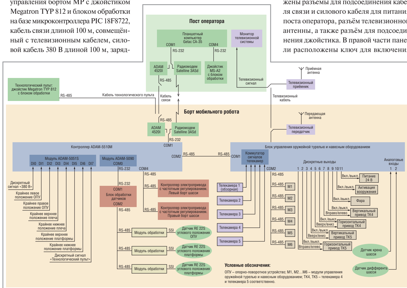
Рис. 2. Структурная схема системы управления МРК-47БТ
