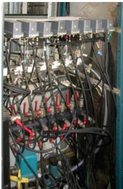
Рис. 4. Шкаф с преобразователями ЭПП и ПЭП
