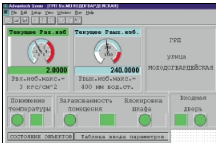
Рис. 8. Отображение телеметрической информации ГРП
