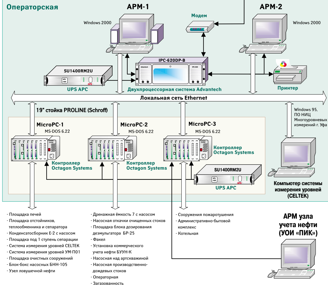
Рис. 5. Типовая структура АСУ ТП подготовки нефти
