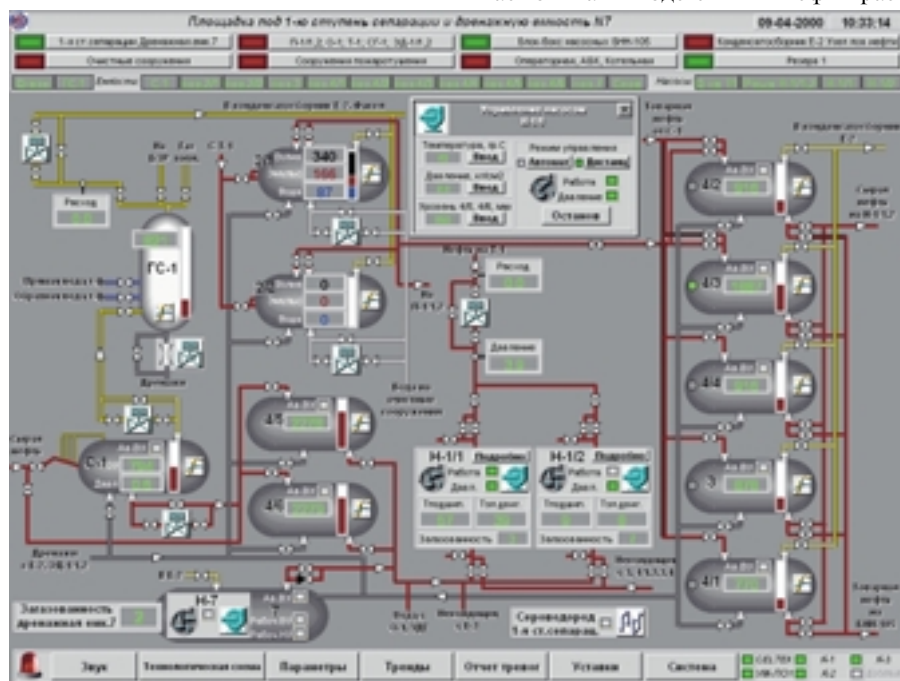
Рис. 9. Пример мнемосхемы АРМ оператора УКПН
