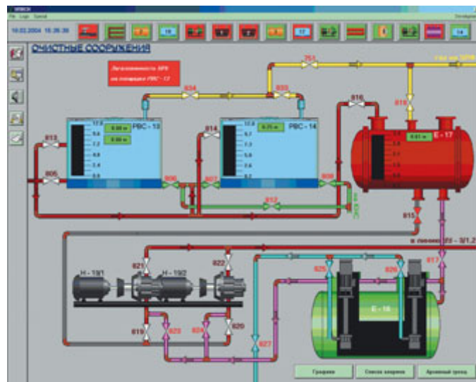
Рис. 7. Мнемосхема «Очистные сооружения»
