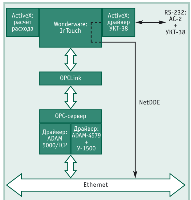
Рис. 3. Структура взаимодействия программного обеспечения
