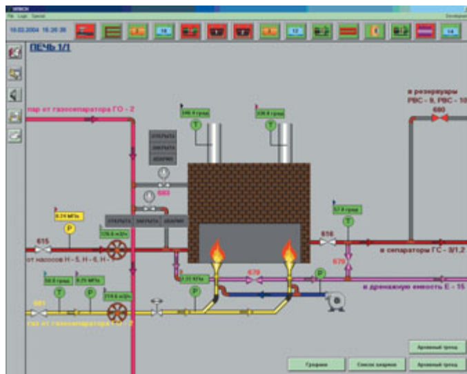
Рис. 6. Мнемосхема «Печь 1/1»
