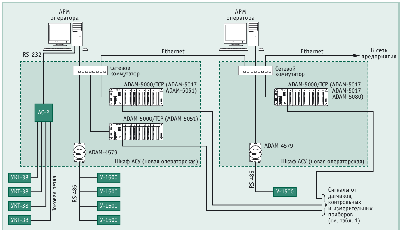
Рис. 2. Структура комплекса технических средств АСУ ТП Акташской УПВСН
