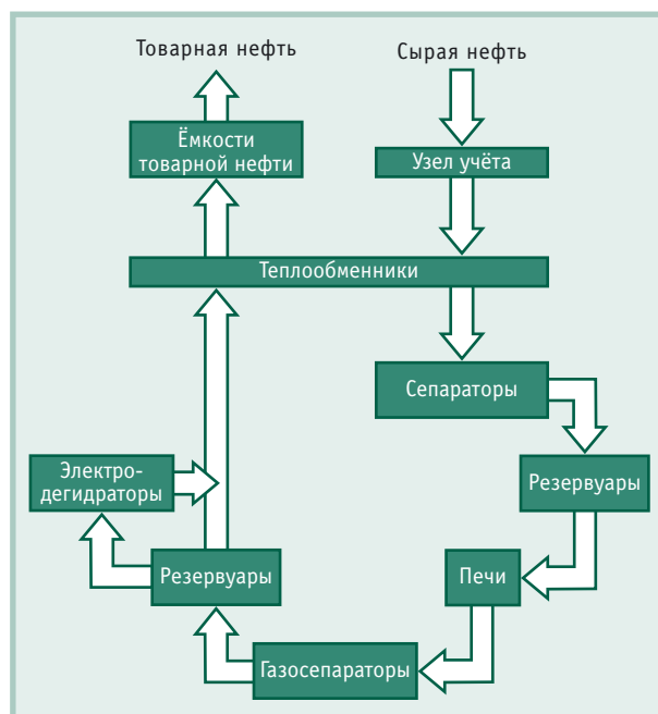
Рис. 1. Схема процесса очистки нефти на УПВСН
