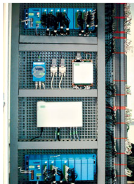
Рис. 5. Шкаф с аппаратурой АСУ ТП в новой операторской
