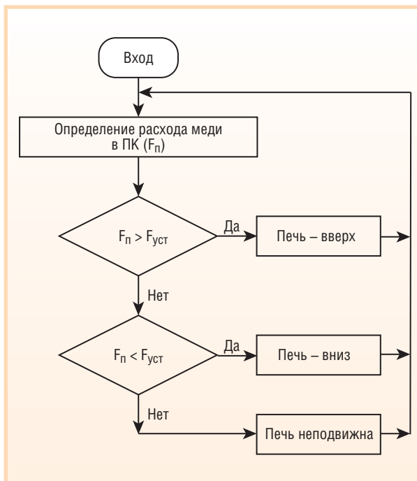
Рис. 8. Упрощенная блок-схема алгоритма управления расходом меди из печи
