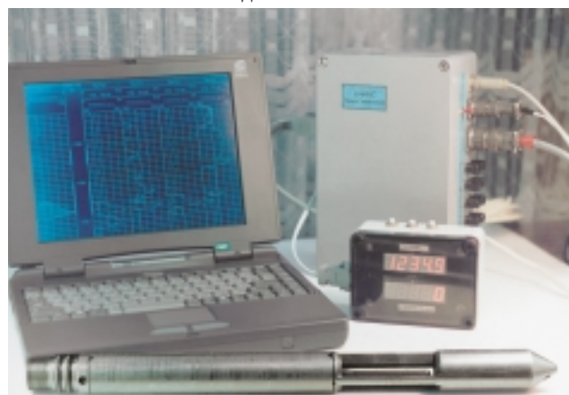
Станция ОНИКС со скважинным прибором
