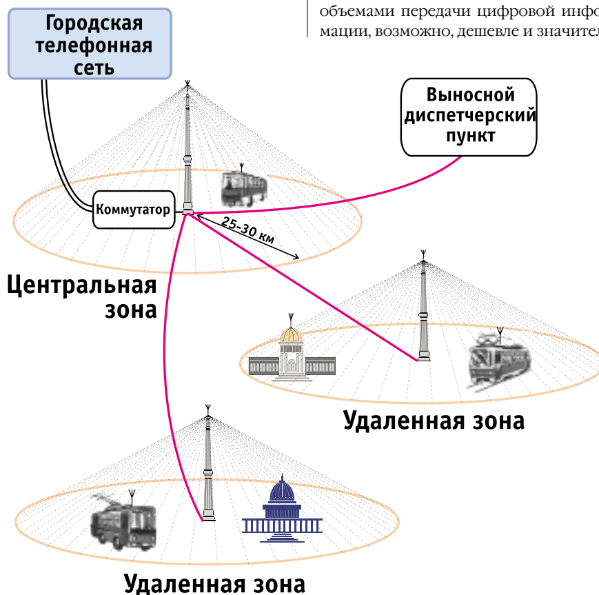
Рис. 2. Транковая система связи
