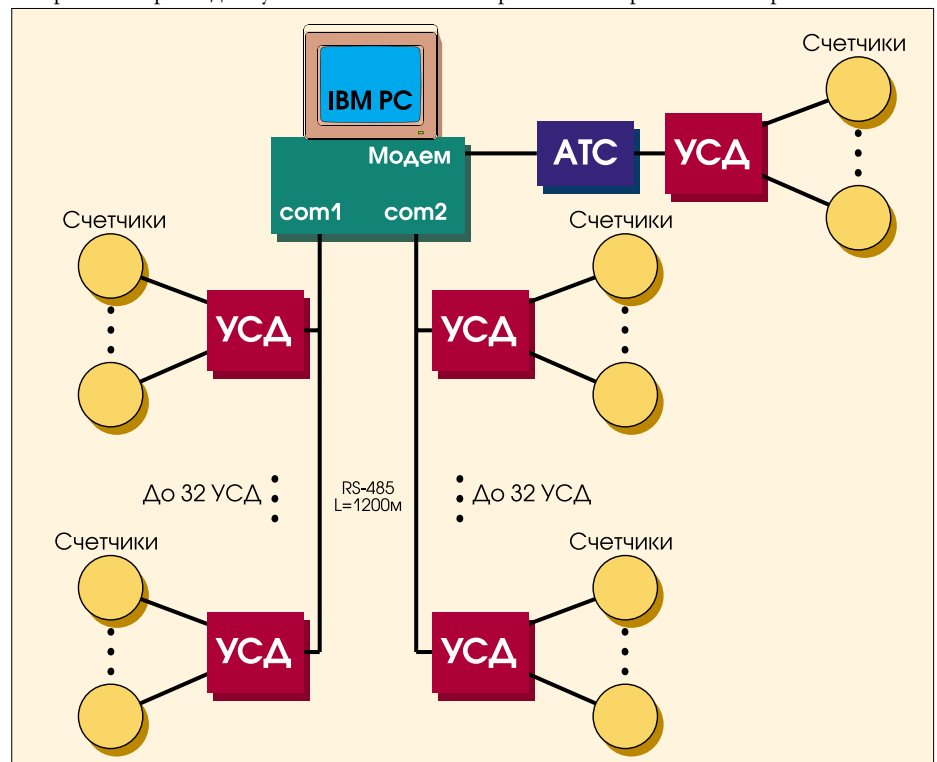
Рис. 2. Структура системы учета электропотребления
