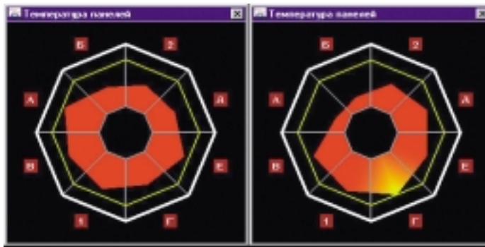
Рис. 9. Распределение температур в топке котла Е-820 при различных регулировках (справа технологически неприемлемый перекос факела)
