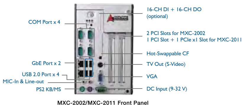
MXC-2002/MXC-2011 Front Panel
